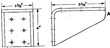
KNEE
